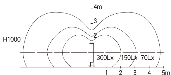
配光曲線断面図
