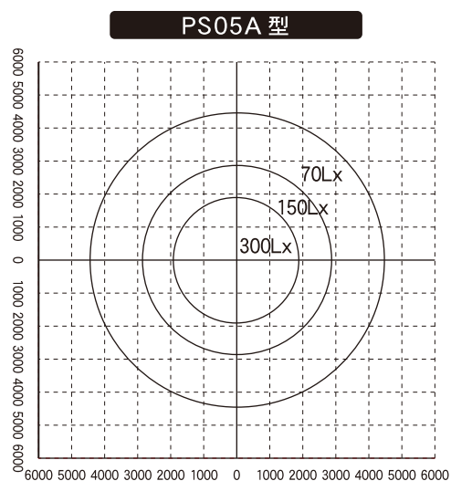
配光曲線図
