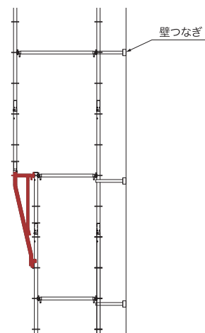
拡幅としての使用時
